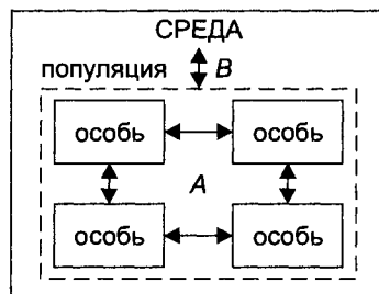
Рис. 3.10. Связи экологической системы для модели 3
