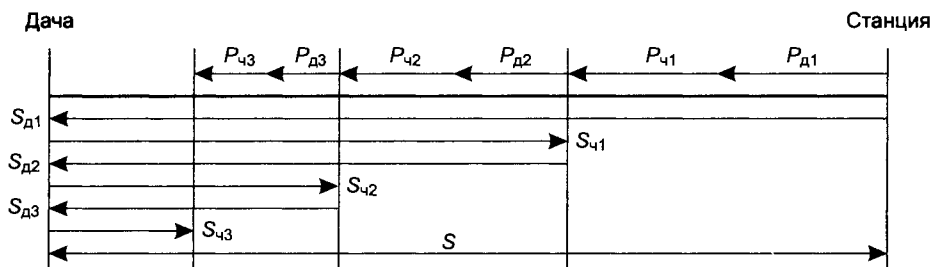
Рис. 3.1. Процесс движения пешехода и собаки
