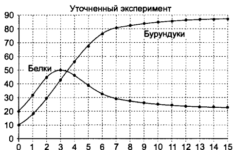
Рис. 3.13. изменения численности популяции при соперничестве видов
