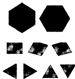
Рис. 1.9. Меню паркета
