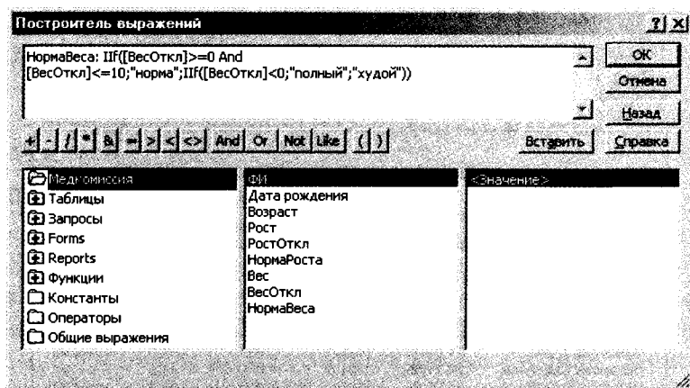
Рис. 4.9. Построитель выражений
